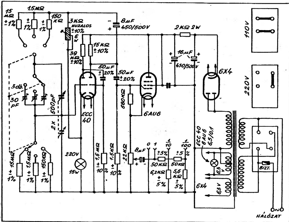
EMG Servotest 1925 típusú
