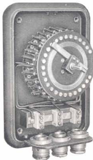
Hangerőszabályzó nyitva.
